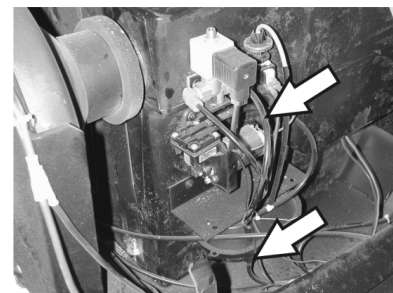
Slangetilkobling for undertrykkpumpe og til undertrykkslange (akkumulator)
