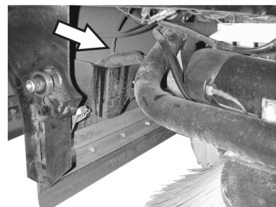
Slangetilkobling for undertrykkslange for senking av sidebørster
