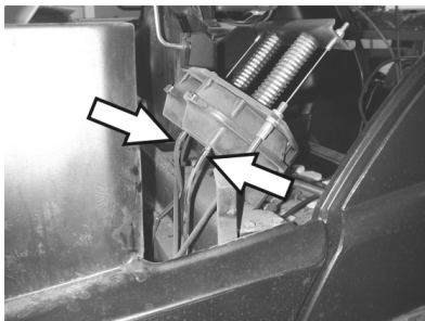
Priklučci crijeva za vakuumsku utičnicu dijela za spuštanje valjaka za metenje
