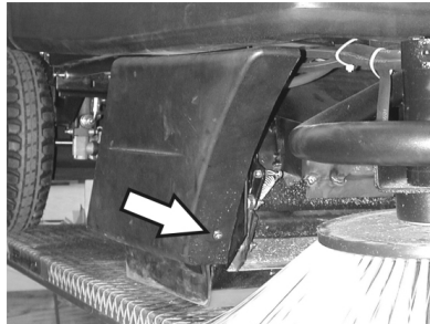
Sļūteņu pieslēgumi slaucītājveltna nolaišanas mehānisma vakuuma kārbai
