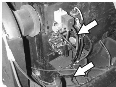
Priklučci crijeva za vakuumsku pumpu i za vakuumsku utičnicu (spremnik)
