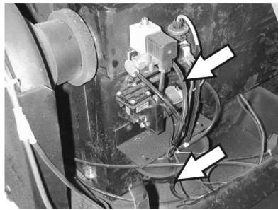
Slangaansluitingen naar de onderdruk-pomp en de onderdrukdoos (reservoir) Instructie: De onderdruk-pomp draait alleen wanneer onderdruk in het systeem opgebouwd wordt. Indien de pomp altijd draait, moet de klantendienst op de hoogte gebracht worden.
