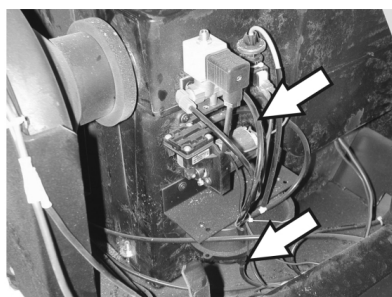
Racorduri de furtun la pompa de subpresiune și la cutia de subpresiune (rezervor) Indicație: Pompa de subpresiune funcționează doar când în cadrul sistemului se generează subpresiune. Dacă pompa funcționează în continuu, contactați serviciul pentru clienți.
